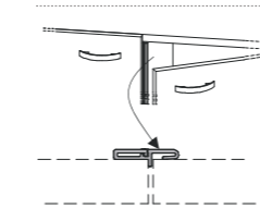
503.CU.PP.01.11 H 79,6 503.CU.PP.01.31 H 124,4 503.CU.PP.01.41 H 159,6 503.CU.PP.01.51 H 204,4 Profilo battiporta parapolvere per contenitori / Dust-proof / door-latch profile for units
